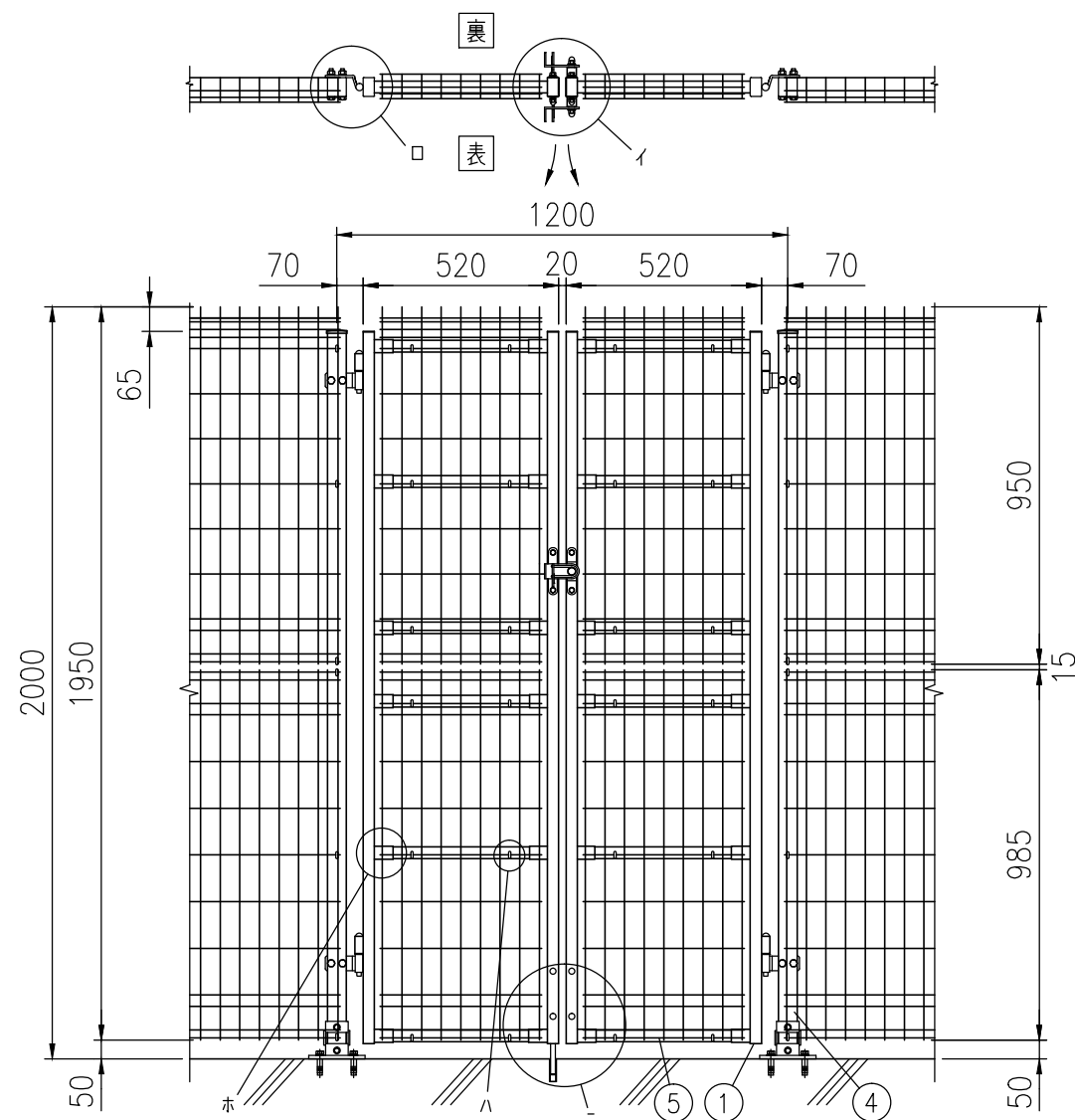
組立図 表開き、落とし棒が裏の時 (1/20) 注> 基礎の大きさは参考寸法です。
