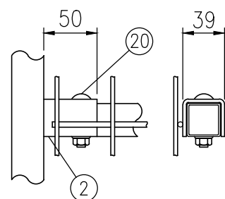
ホ部詳細図 (1/5)
