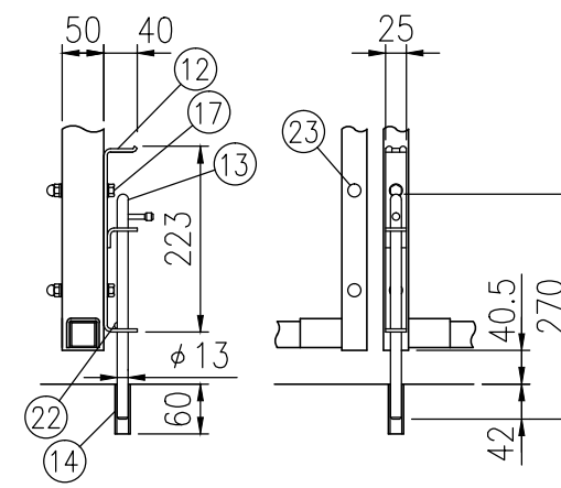
ニ部詳細図 (1/10)
