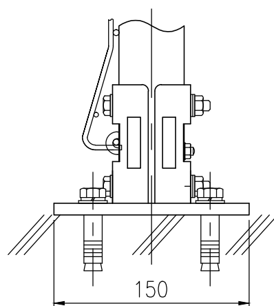
ベースプレート詳細図 (1/4)
