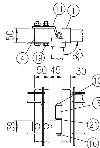
ロ部詳細図 (1/8)
