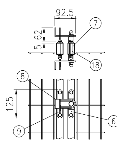
イ部詳細図 (1/10)
