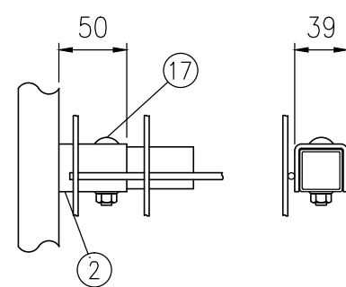
ニ部詳細図 (1/5)
