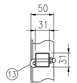
ハ部詳細図 (1/5)
