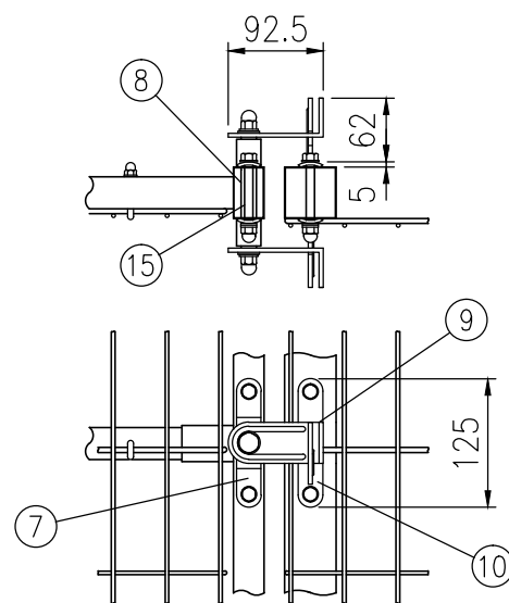
イ部詳細図 (1/8)
