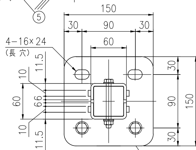
イ部詳細図 (1/8)
