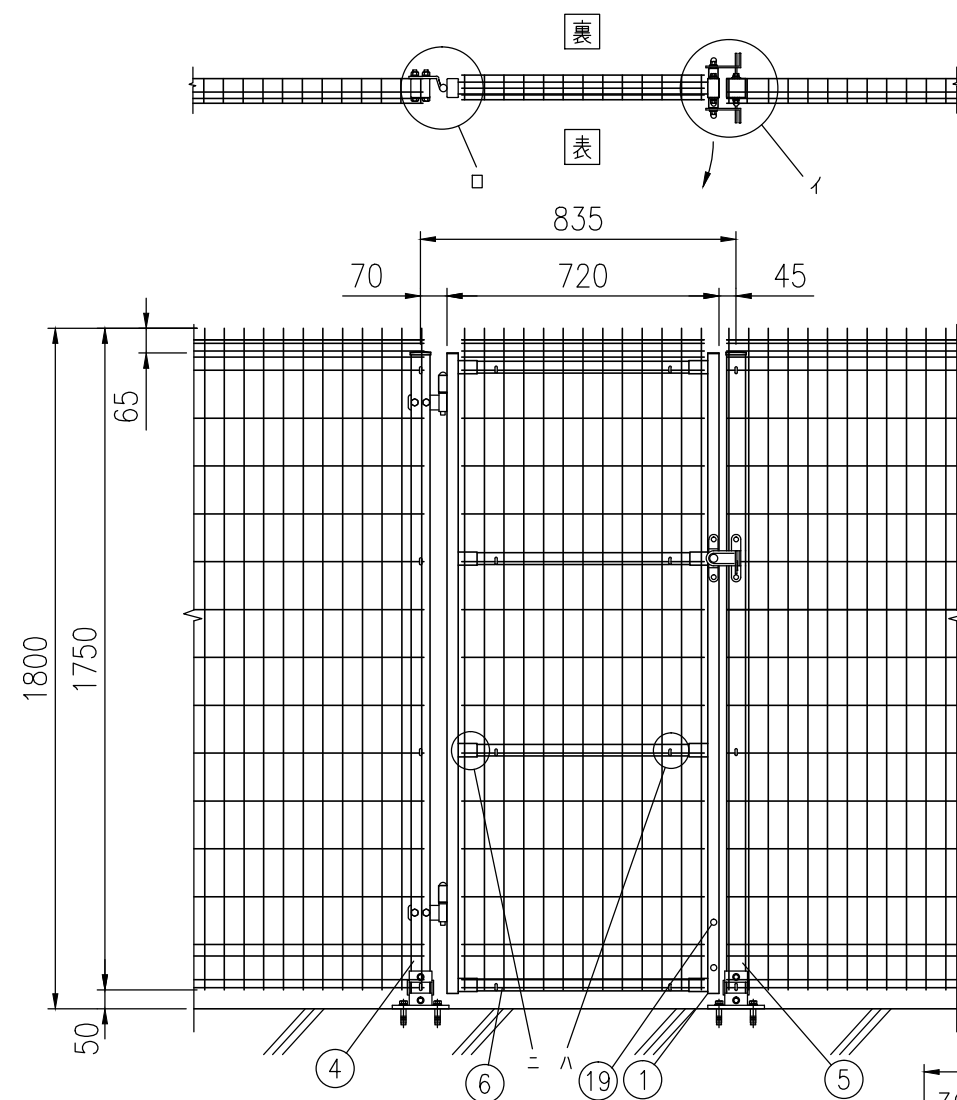
組立図 吊元が左、表開き (1/20) 注>基礎の大きさは参考寸法です。
