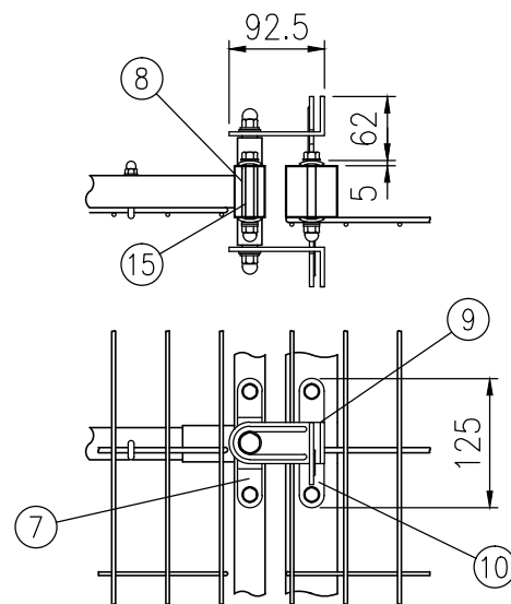
イ部詳細図 (1/8)
