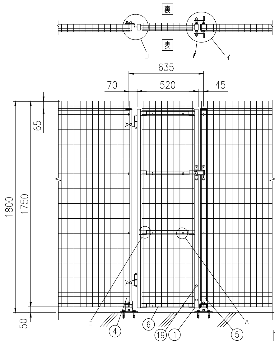
組立図 吊元が左、表開き (1/20) 注>基礎の大きさは参考寸法です。
