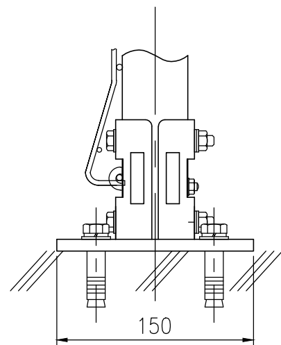
ベースプレート詳細図 (1/4)
