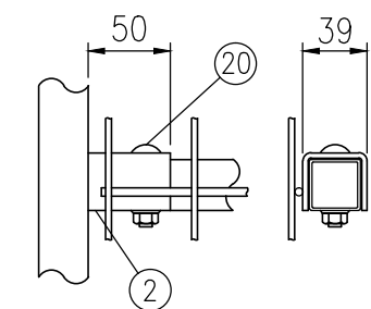
ホ部詳細図 (1/5)
