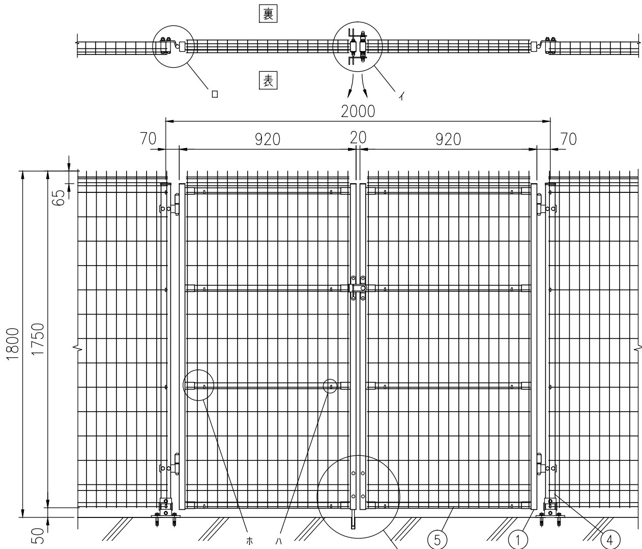
組立図 表開き、落とし棒が裏の時 (1/20) 注> 基礎の大きさは参考寸法です。
