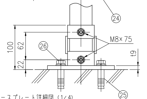
ベースプレート詳細図 (1/4)
