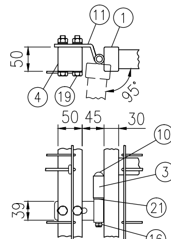
ロ部詳細図 (1/8)
