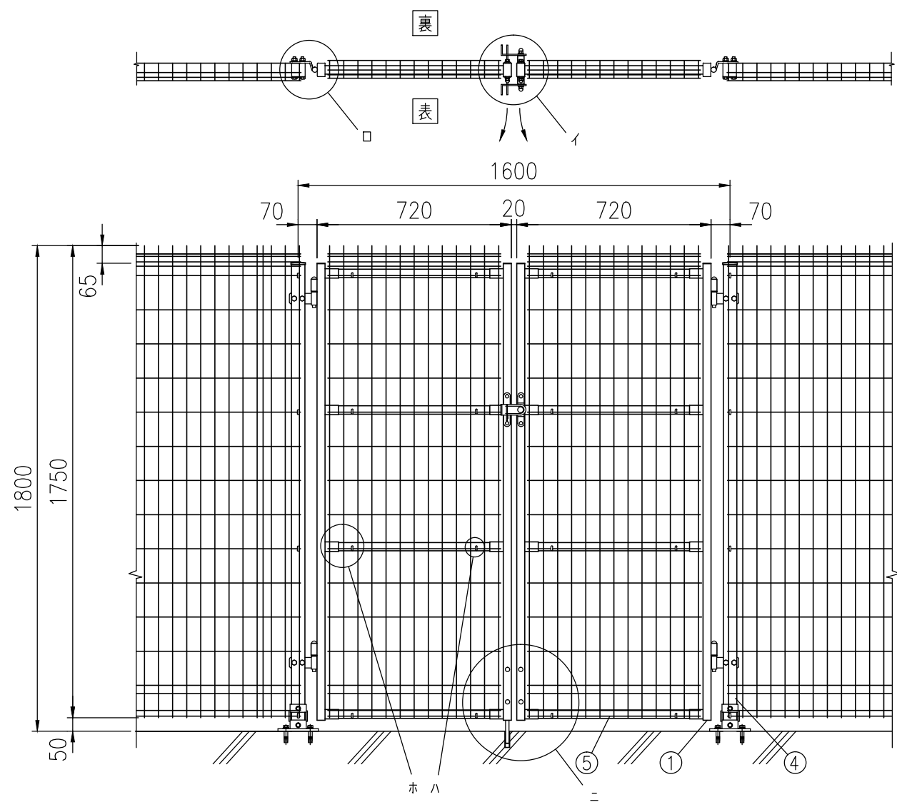
組立図 表開き、落とし棒が裏の時 (1/20) 注>基礎の大きさは参考寸法です。
