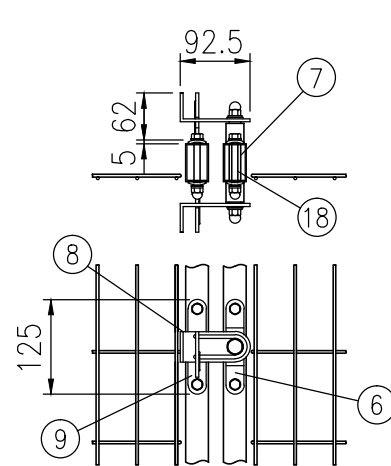
イ部詳細図 (1/10)
