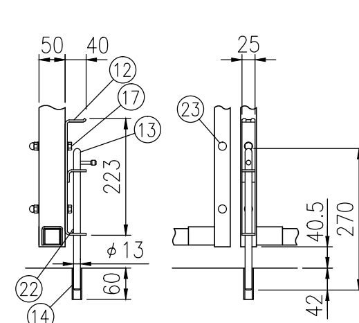
ニ部詳細図 (1/10)
