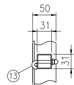
ハ部詳細図 (1/5)
