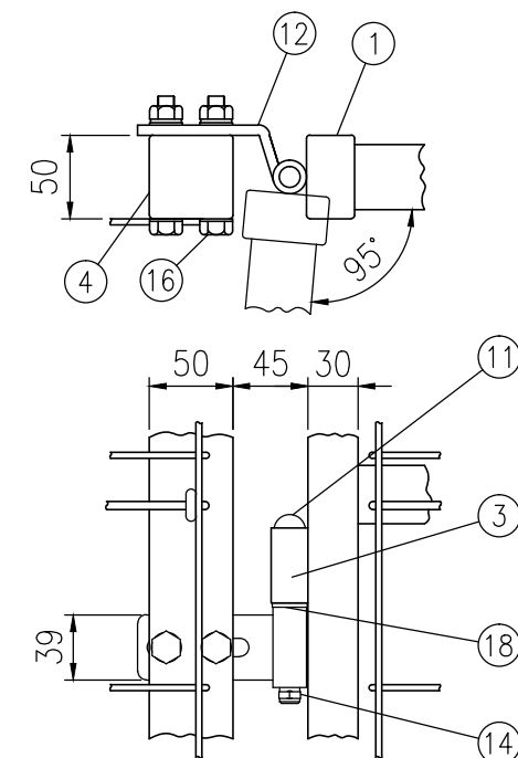
ロ部詳細図 (1/5)
