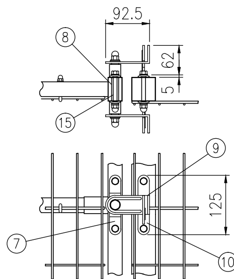
イ部詳細図 (1/8)
