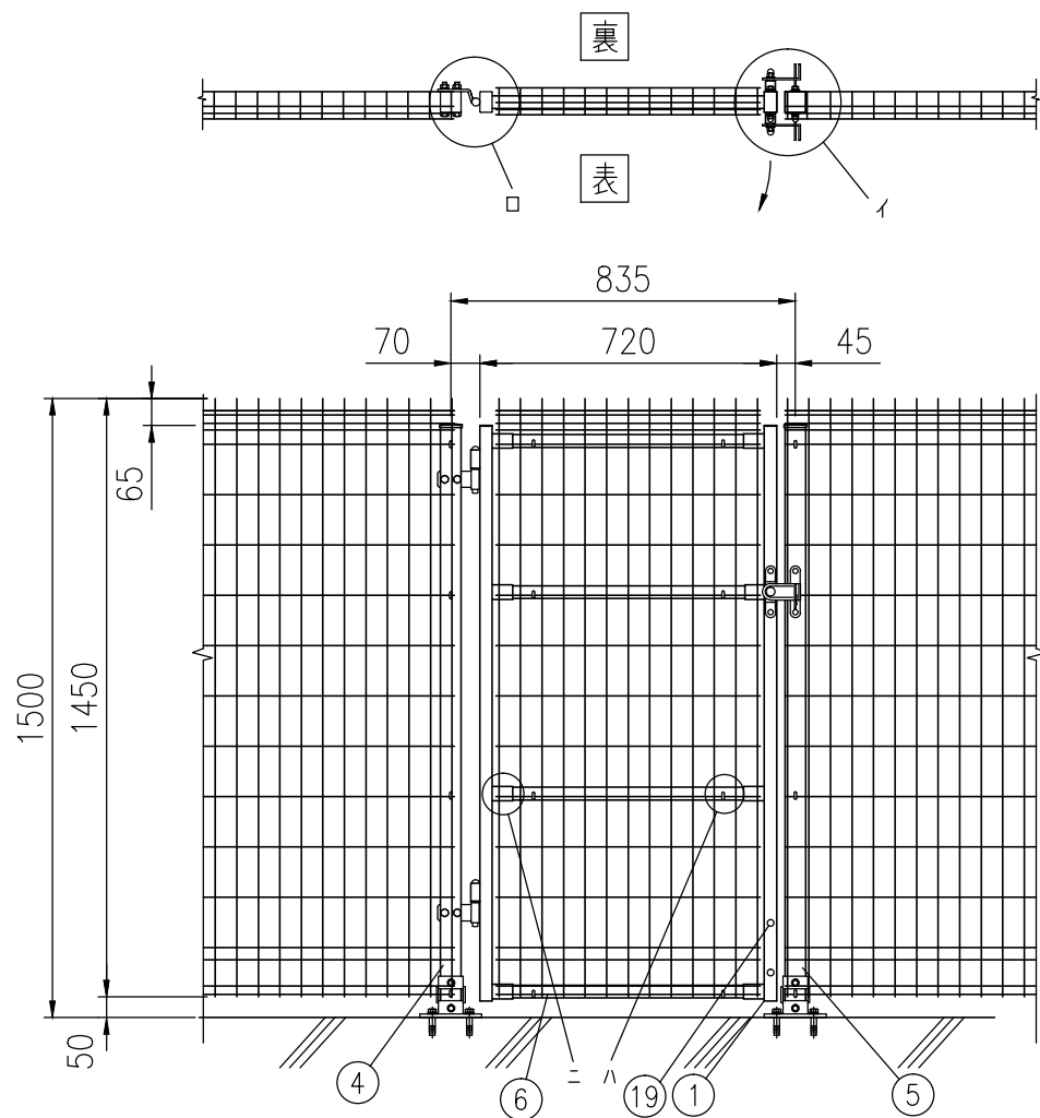
組立図 吊元が左、表開き (1/20)
