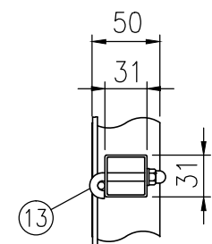
H部詳細図 (1/5)
