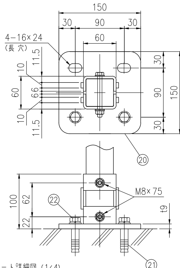
ベースプレート詳細図 (1/4)
