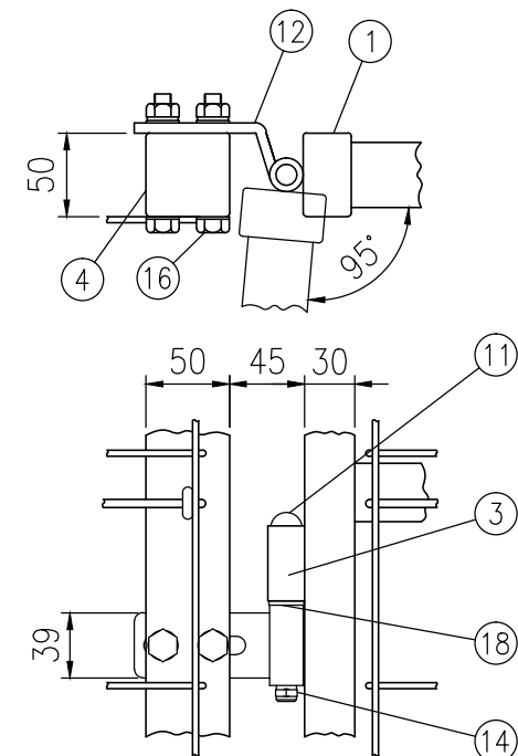
K部詳細図 (1/5)
