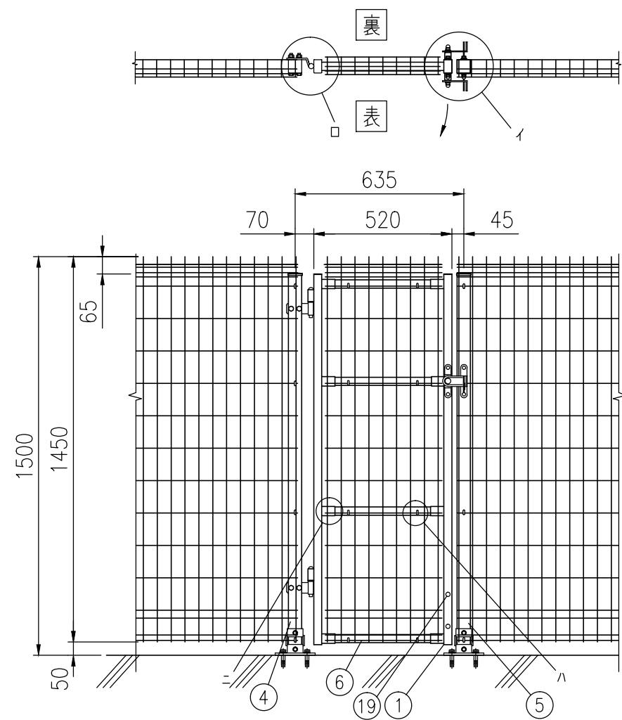
組立図 吊元が左、表開き (1/20)
