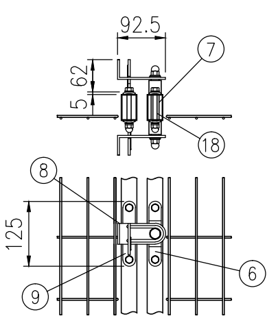
イ部詳細図（1/10）
