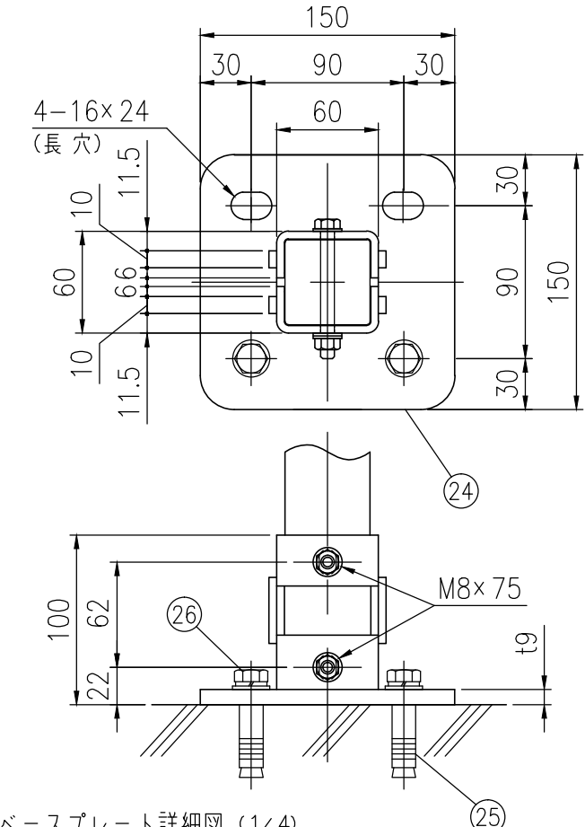
ベースプレート詳細図（1/4）
