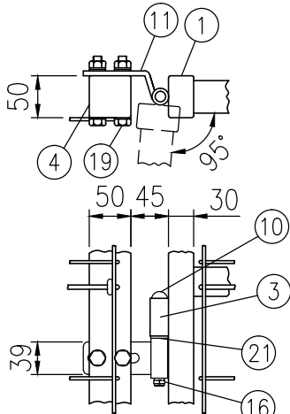
ロ部詳細図（1/8）
