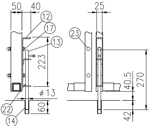
ニ部詳細図（1/10）
