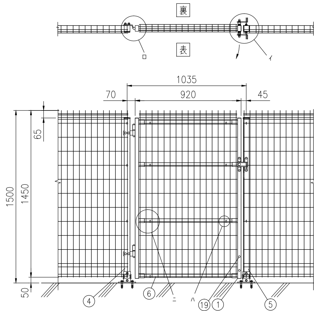
組立図 吊元が左、表開き (1/20)
