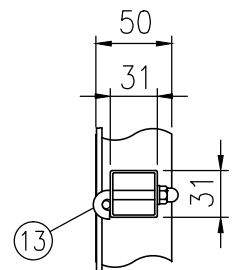
ハ部詳細図 (1/5)
