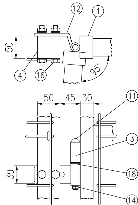
ロ部詳細図 (1/5)
