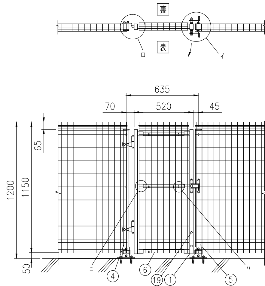
組立図 吊元が左、表開き (1/20) 注>基礎の大きさは参考寸法です。
