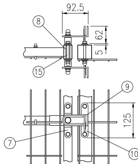
イ部詳細図 (1/8)
