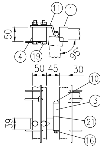
ロ部詳細図 (1/8)
