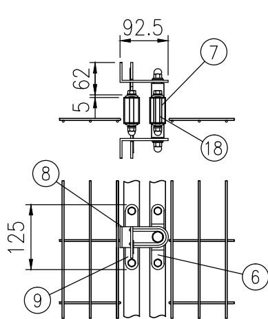
イ部詳細図 (1/10)
