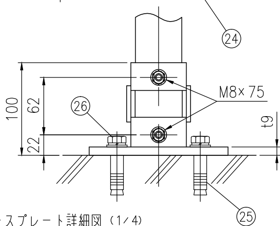
ベースプレート詳細図 (1/4)
