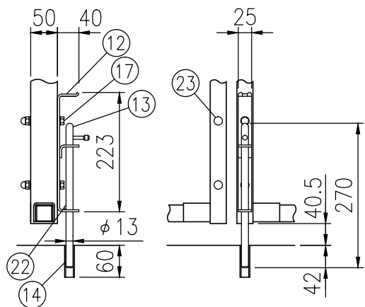
二部詳細図 (1/10)
