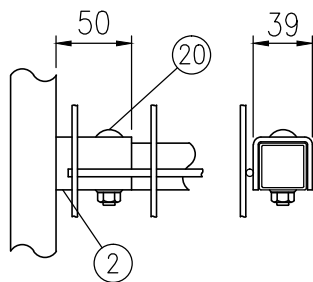
ホ部詳細図 (1/5)
