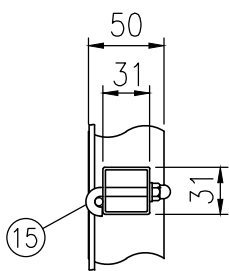
ハ部詳細図 (1/5)
