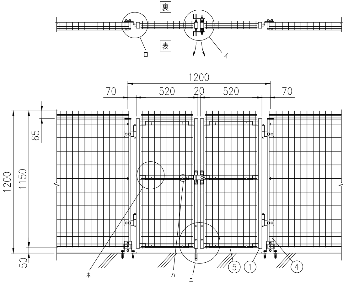
組立図 表開き、落とし棒が裏の時（1/20） 注> 基礎の大きさは参考寸法です。
