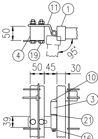
ロ部詳細図（1/8）
