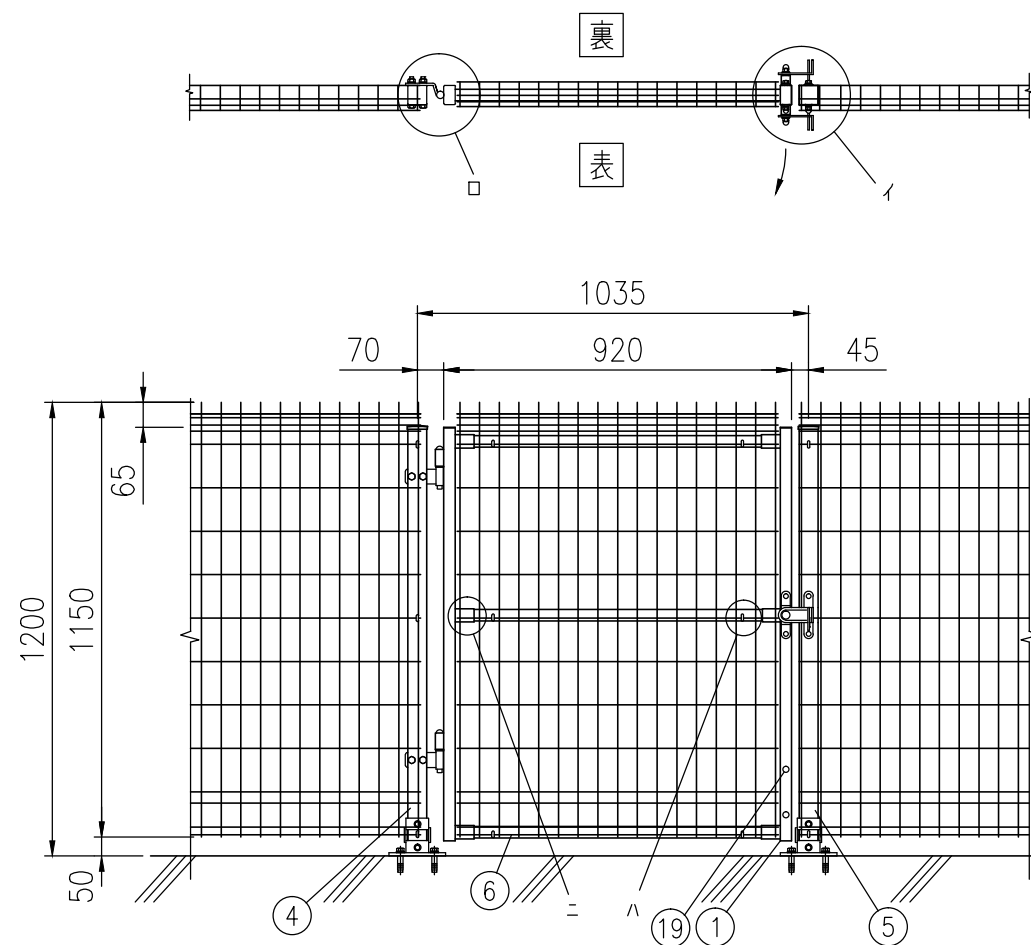
組立図 吊元が左、表開き (1/20)
