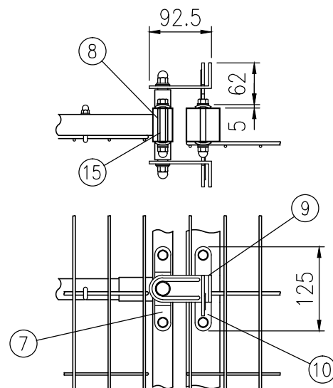
イ部詳細図 (1/8)
