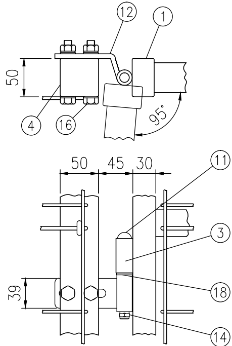
ロ部詳細図 (1/5)
