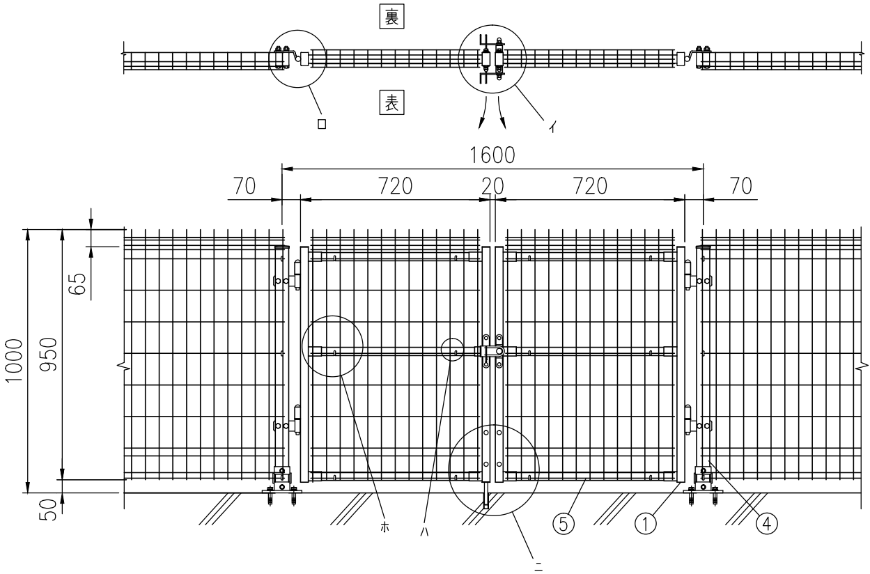
組立図 表開き、落とし棒が裏の時（1/20） 注＞基礎の大きさは参考寸法です。
