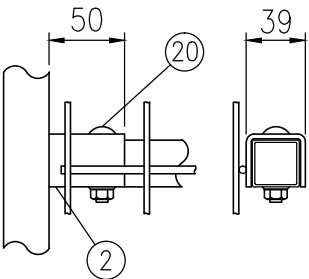
ホ部詳細図（1/5）
