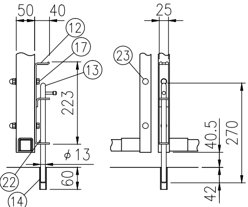
ニ部詳細図（1/10）
