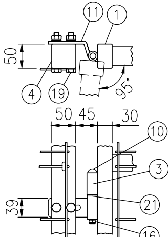
II部詳細図（1/8）
