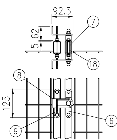
I部詳細図（1/10）
