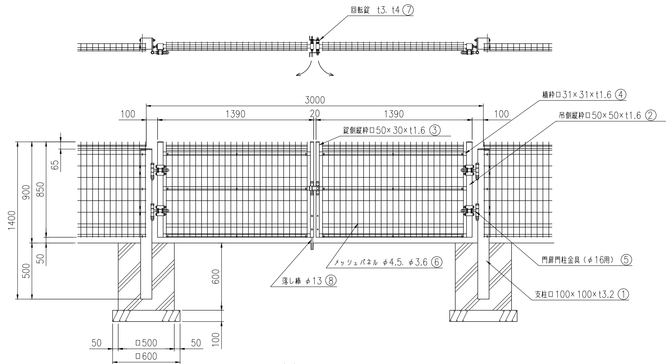
組立図（1 / 20） 基礎の大きさは、参考寸法です。
