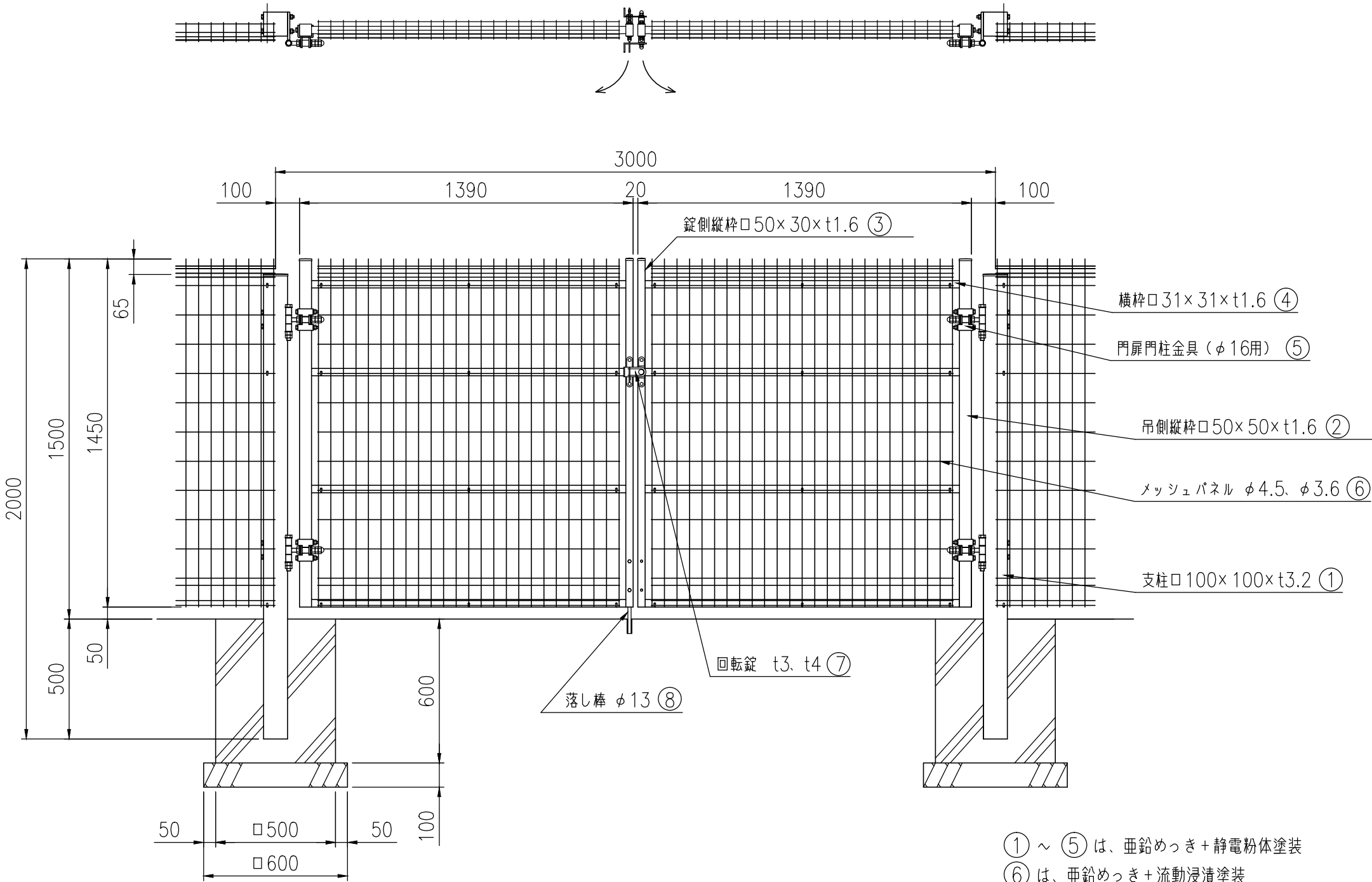
組立図（1／20） 基礎の大きさは、参考寸法です。
