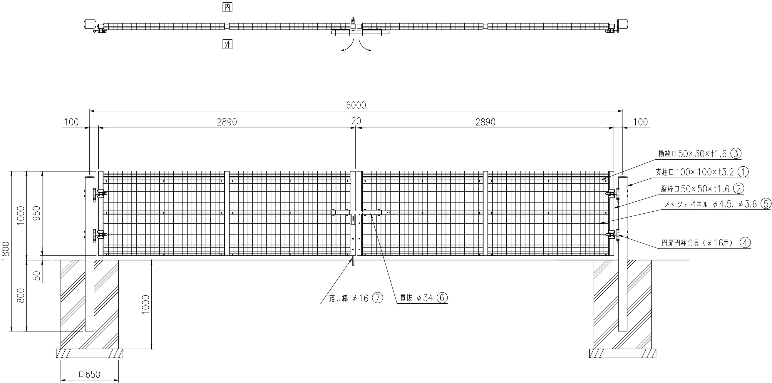
組立図(1/25) 基礎の大きさは、参考寸法です。
