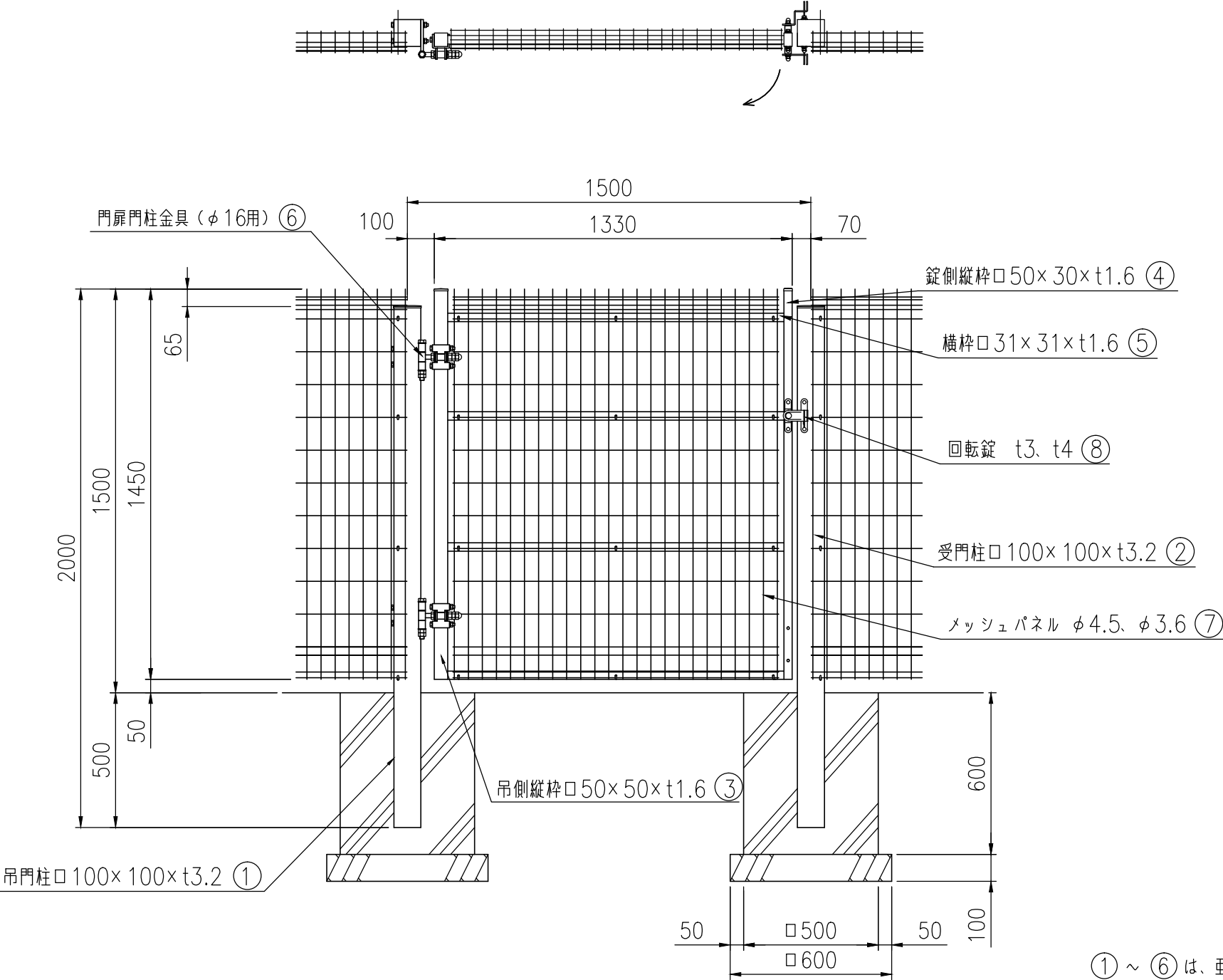
組立図（1／20） 基礎の大きさは、参考寸法です。
