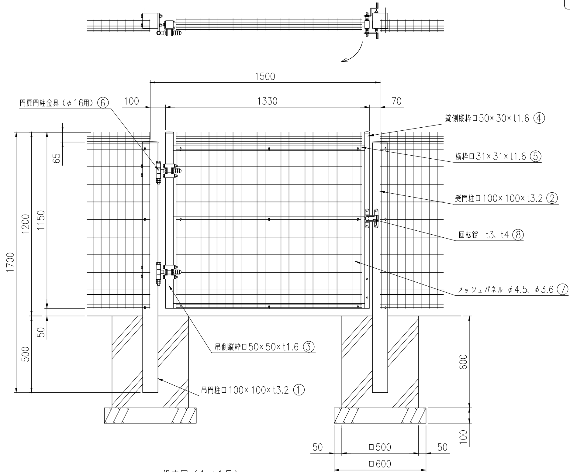
組立図 (1 / 15) 基礎の大きさは、参考寸法です。
