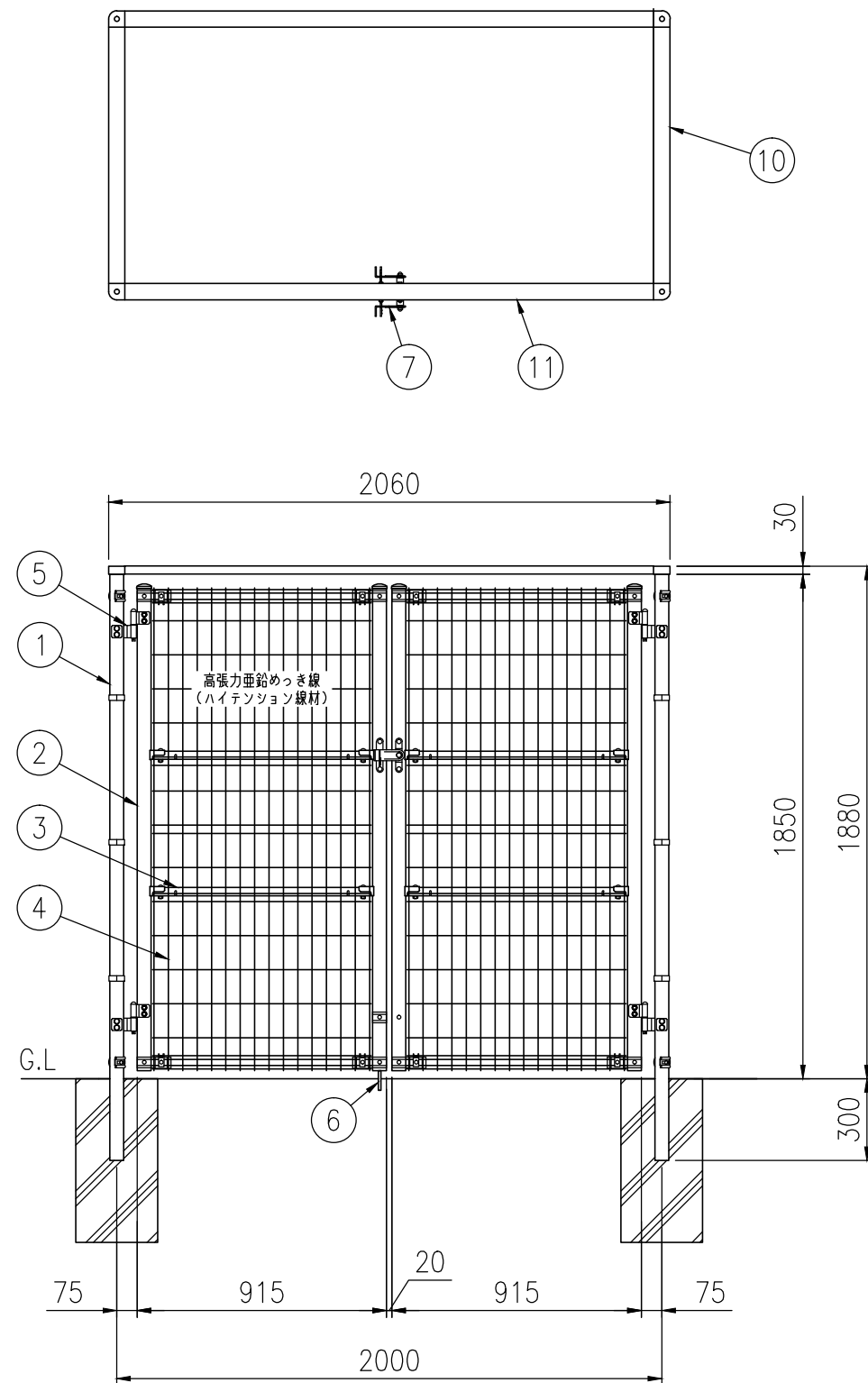
組立図 (S=1/25)
