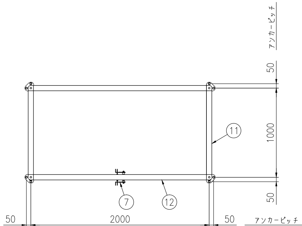
組立図 (S=1/25)
