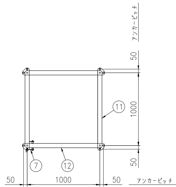
組立図 (S=1/25)
