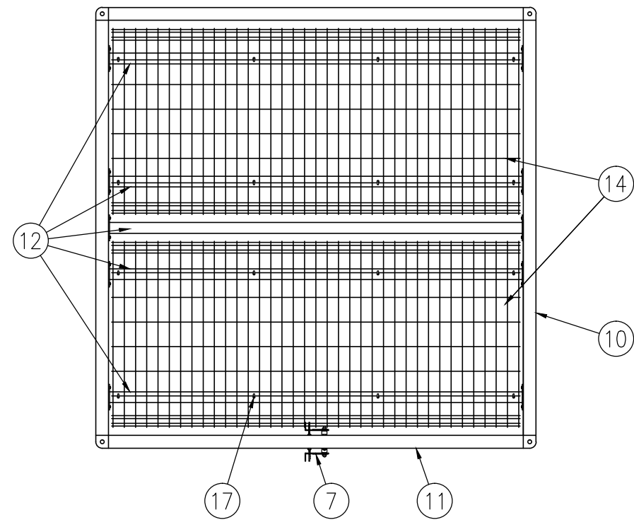
組立図 (S=1/25)
