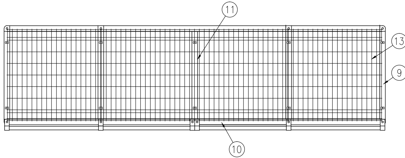
組立図 (S=1/25)
