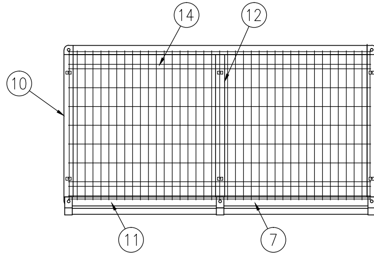
組立図 (S=1/25)
