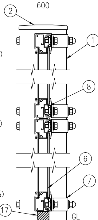
E部 詳細図 (1/5)
