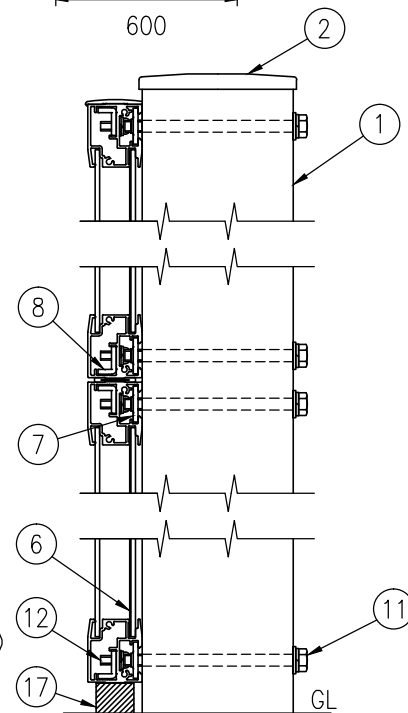
E部 詳細図 (1/5)
