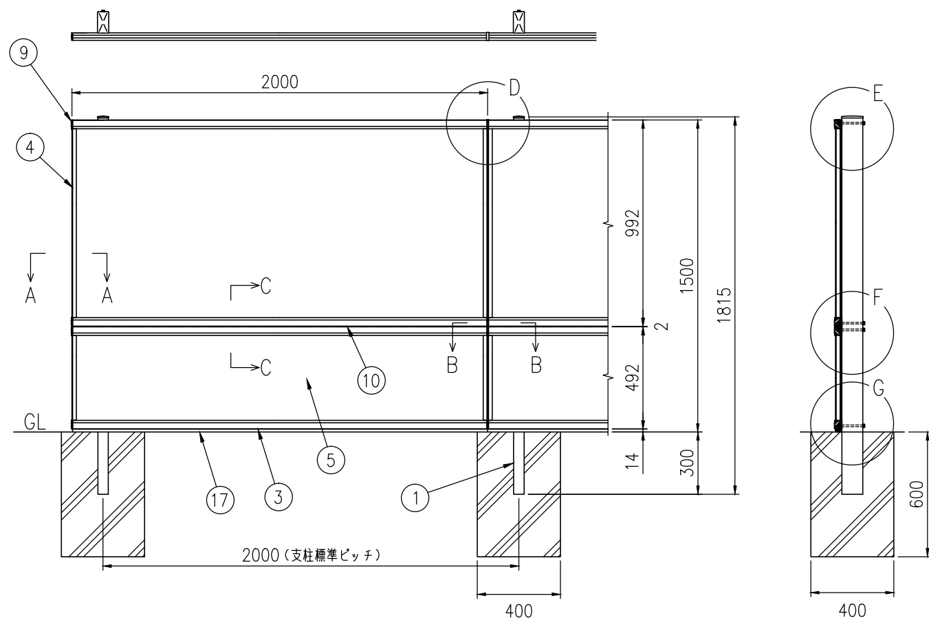
組立図 (1/25)
