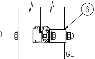
G部 詳細図 (1/5)
