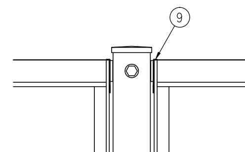
D部 詳細図 (1/5)
