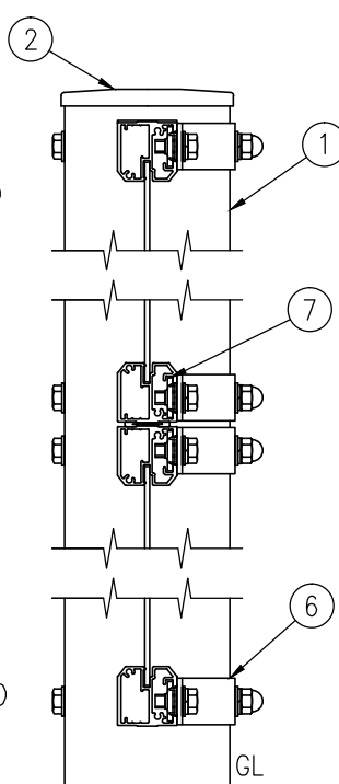
E部 詳細図 (1/5)
