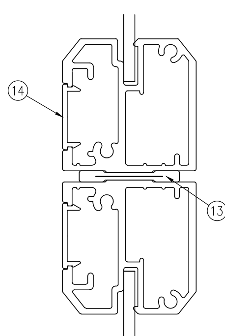
C-C 断面図 (1/1)
