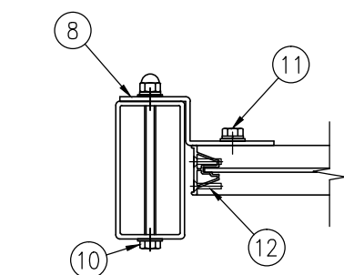
A-A断面図 (1/5)
