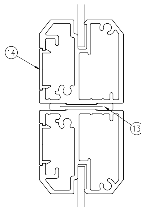
C-C断面図 (1/1)
