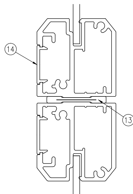
C-C 断面図 (1/1)
