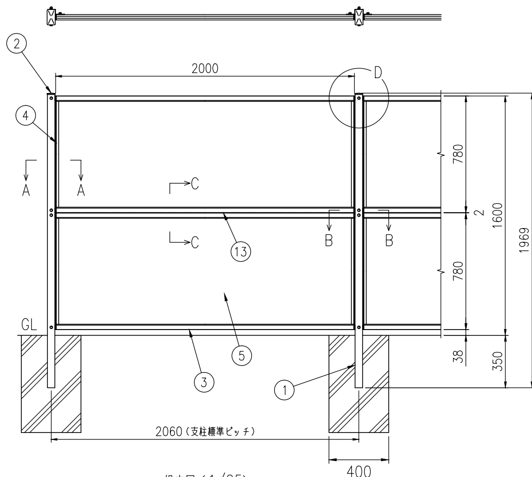
組立図 (1/25)
