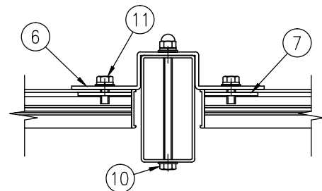
B-B 断面図 (1/5)
