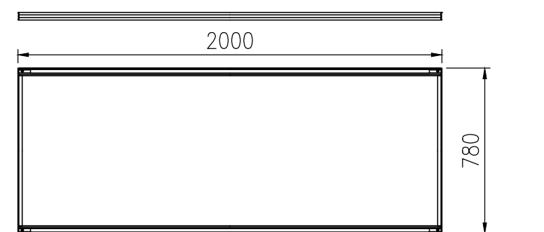
パネル (H800) 詳細図 (1/25)
