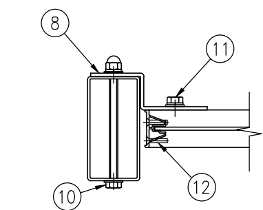
A-A 断面図 (1/5)
