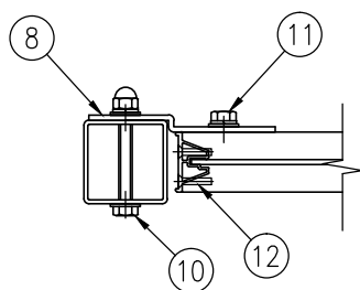
A-A 断面図 (1/5)
