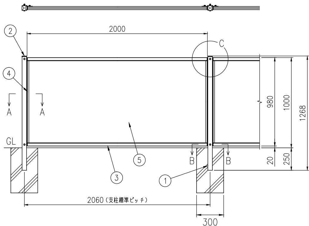
組立図 (1/25)
