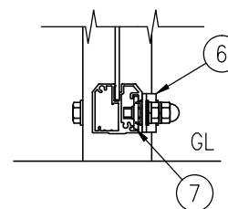
E部 詳細図 (1/5)
