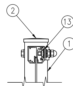
D部 詳細図 (1/5)
