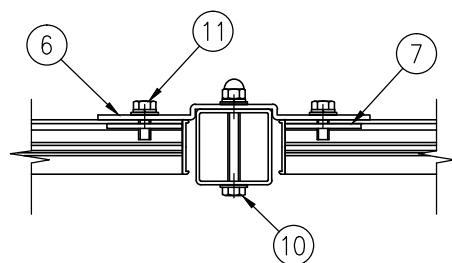
B-B 断面図 (1/5)
