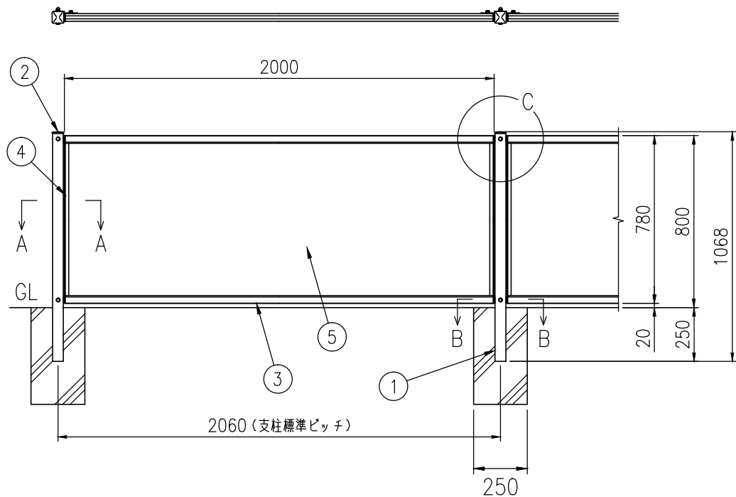
組立図 (1/25)
