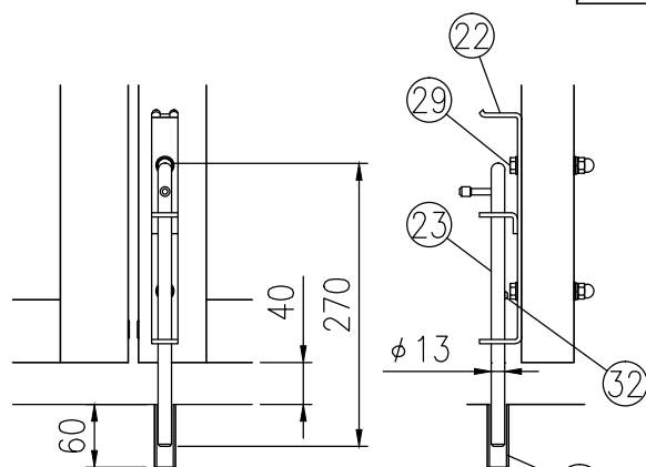
組立図 (1/20) 表開きの時 注) 基礎の大きさは参考寸法です。
