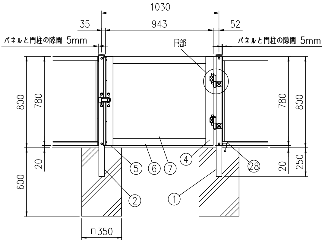
組立図 (1/20)
