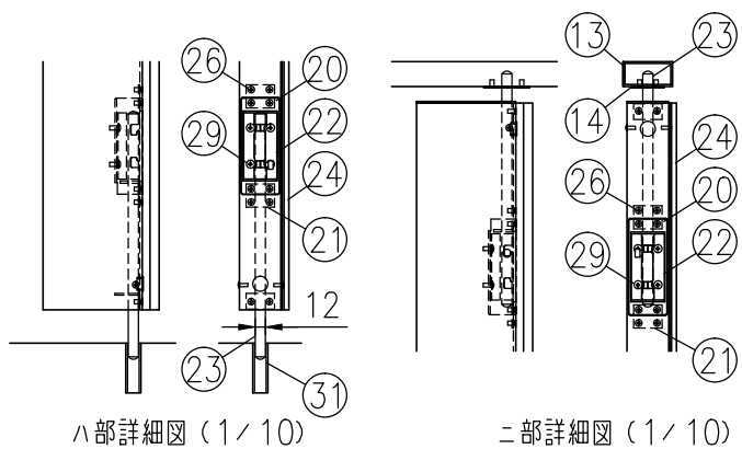
ハ部詳細図 (1/10)
