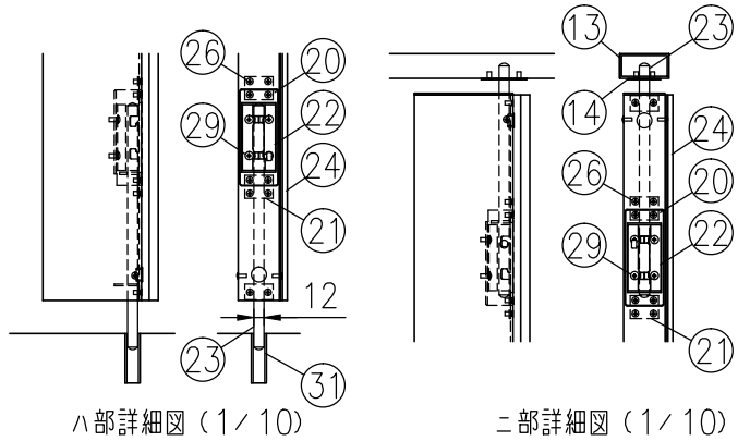
ハ部詳細図 (1/10)
