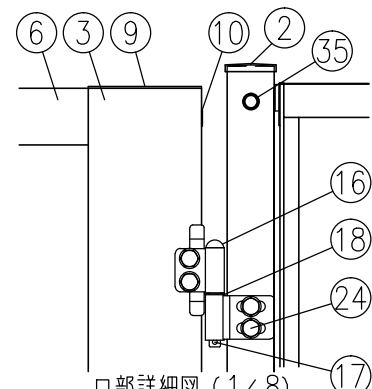
I部分詳細図 (1/8)
