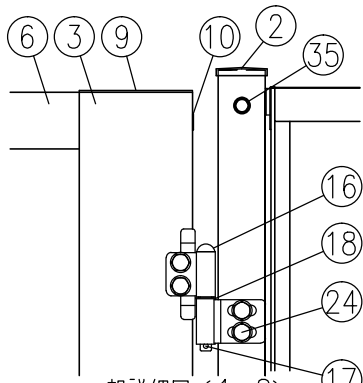
ロ部詳細図 (1/8)
