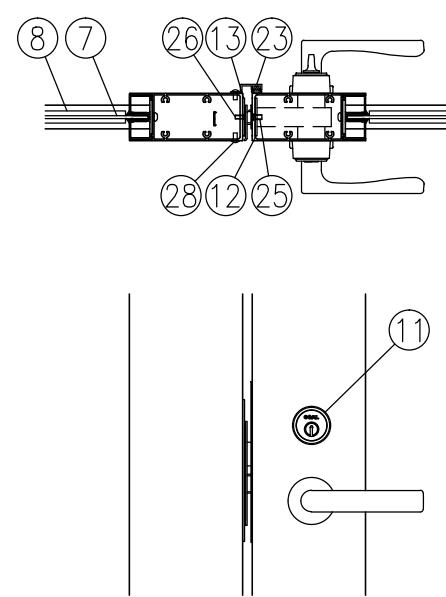
イ部詳細図 (1/8)
