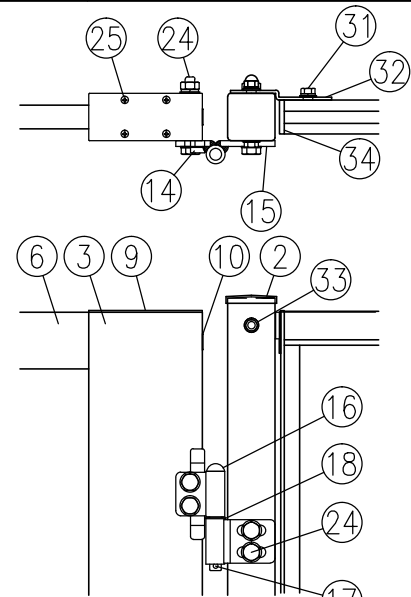
ロ部詳細図 (1/8)
