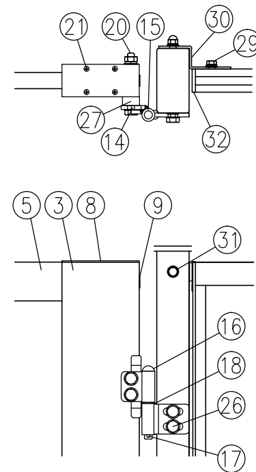
□部詳細図 (1/8)
