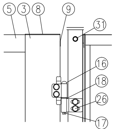
□部詳細図 (1/8)
