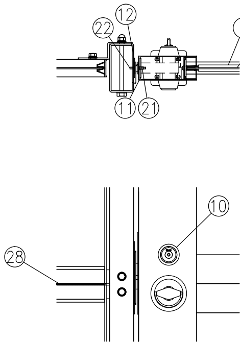
イ部詳細図 (1/8)
