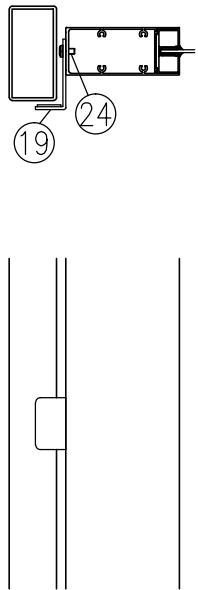
ハ部詳細図 (1/8)
