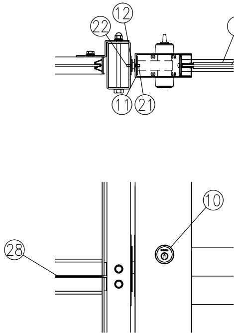
イ部詳細図 (1/8)
