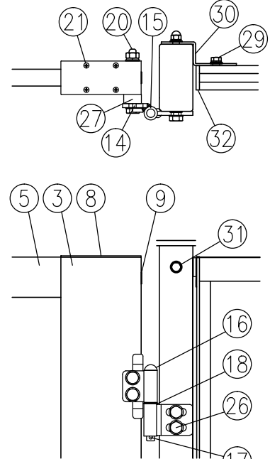
ロ部詳細図 (1/8)
