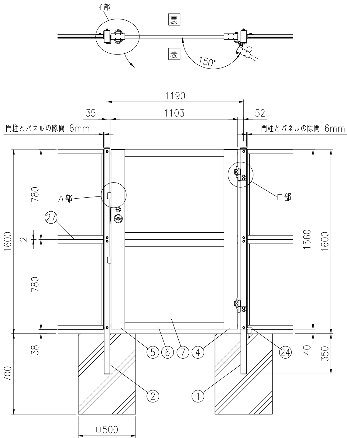
組立図 (1/20)
